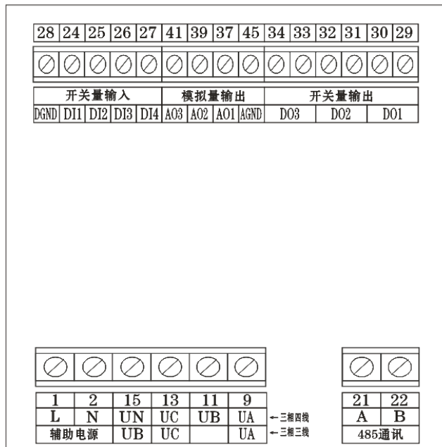
120/96三相电压表
