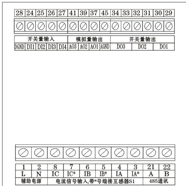
120/96三相电流表
