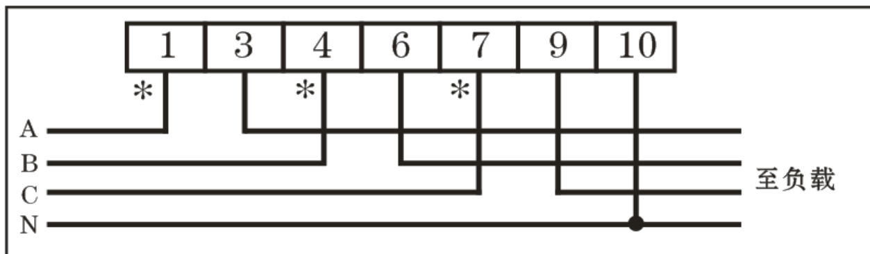
三相四线，直接式（电压 3X220/380V，电流 \geq 3 \times 5 (20) A）；*号端，为进线端
