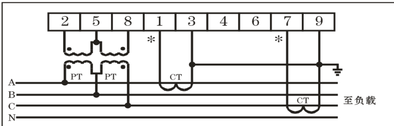
三相三线，电流，电压互感式（电压 3X100V，电流 3X1.5 (6) A)；*号端，为电流进线端
