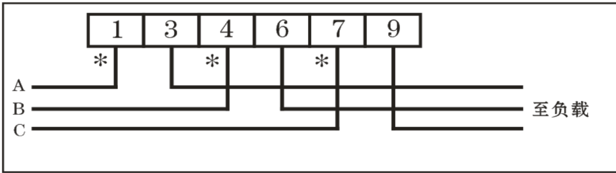
三相三线，直接式（电压 3X220/380V，电流 \geq 3 \times 5 (20) A)；*号端，为进线端
