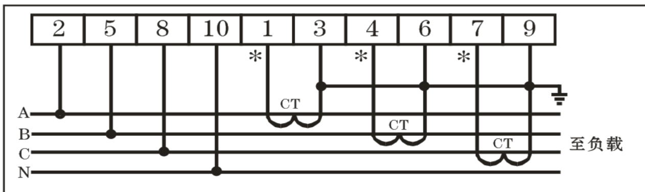
三相四线，电流互感器式（电压 3X220/380V，电流 3 \times 1.5 (6) A）；*号端，为电流进线端
