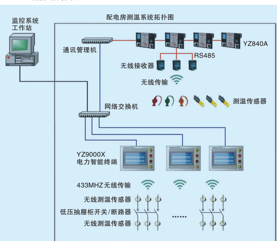
珠海松下马达有限公司无线测温改造工程
